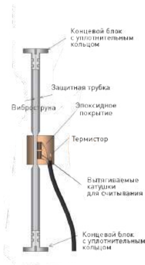
СХЕМА ДАТЧИКА SG4
