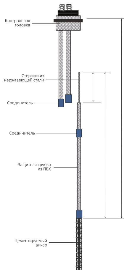
СХЕМА ДАТЧИКА ISSO-EX3-6
