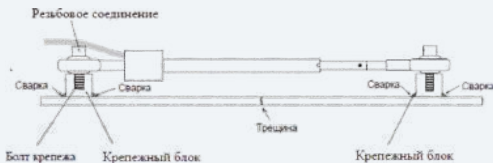
СХЕМА МОНТАЖА ISSO-CR
