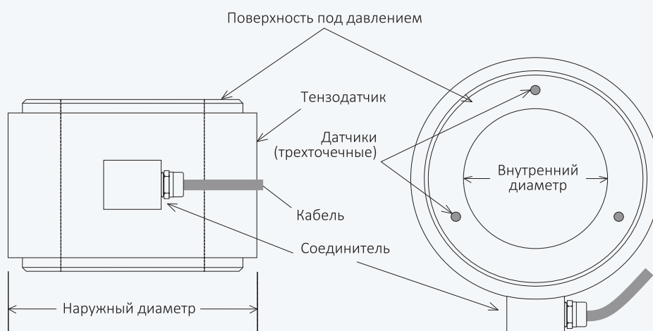
СХЕМА ДАТЧИКА ISSO-LC
