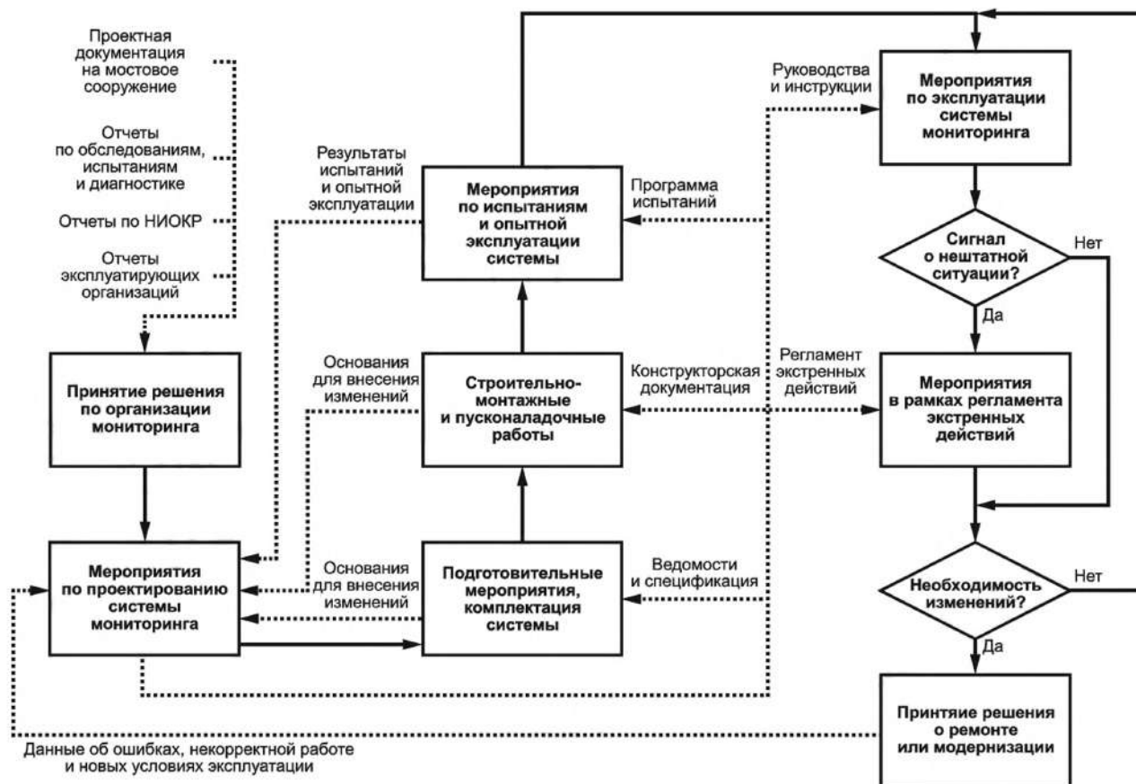
Рисунок 4 — Блок-схема мероприятий по организации системы мониторинга при эксплуатации мостового сооружения
