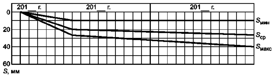
Рисунок Б.4 — График развития перемещений
