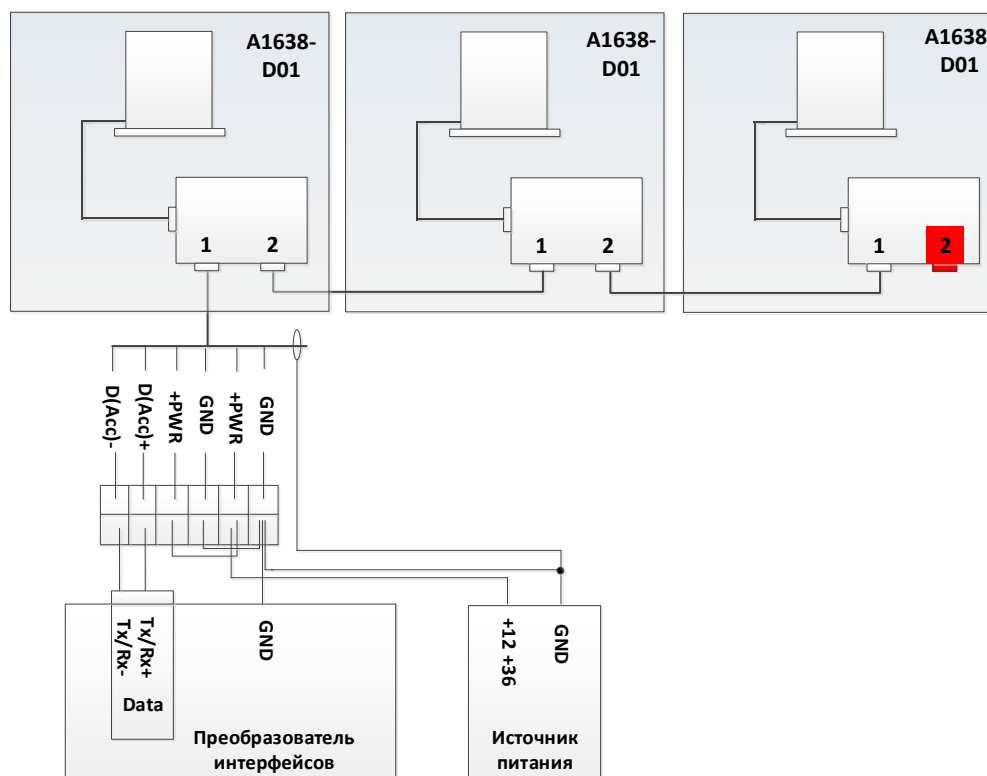
Рисунок 2 – Подключение сейсмоприемников A1638-D01 в измерительную линию
